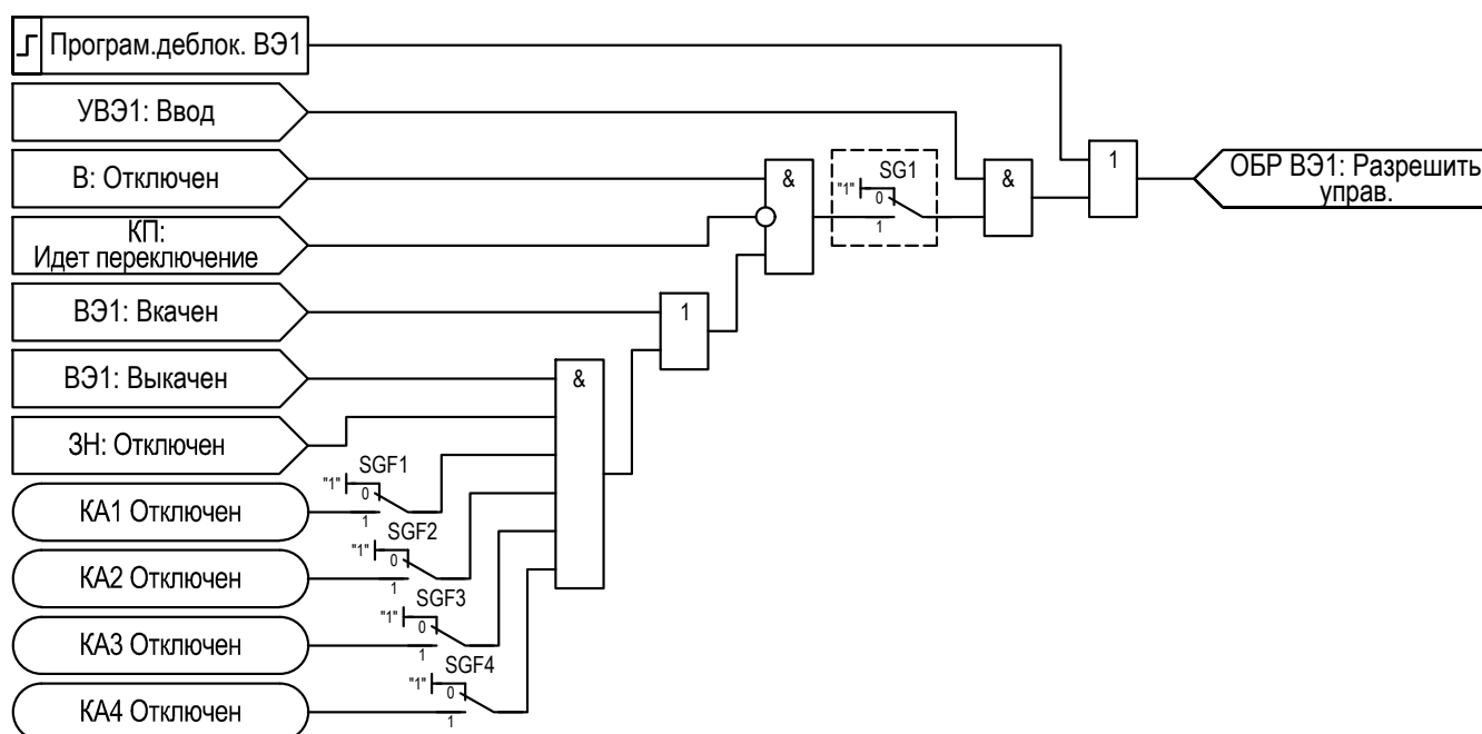
Рисунок 2.53 – Функциональная схема «ОБР ВЭ1»
