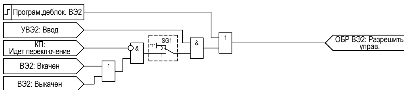
Рисунок 2.54 – Функциональная схема «ОБР ВЭ2»
